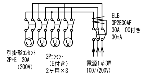
結線図
